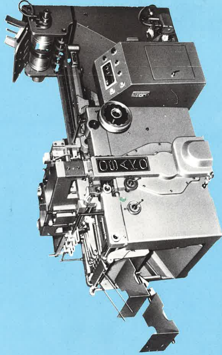
OTF型自動給紙付三方断截機正面図
